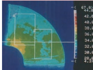
U-ブリッドエルボカバー (当社製品)
