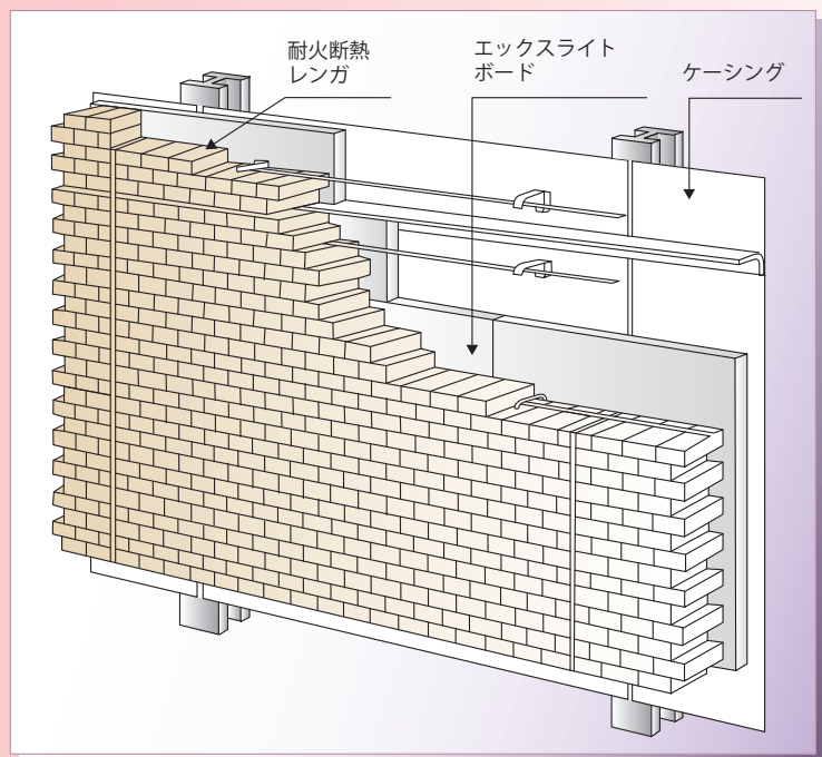
炉壁 / レンガ・エキスライトボード組み合わせ施工例
